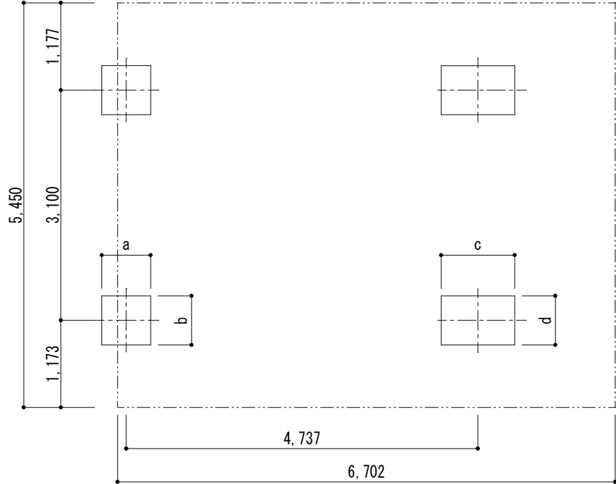
■ 基礎配置図
